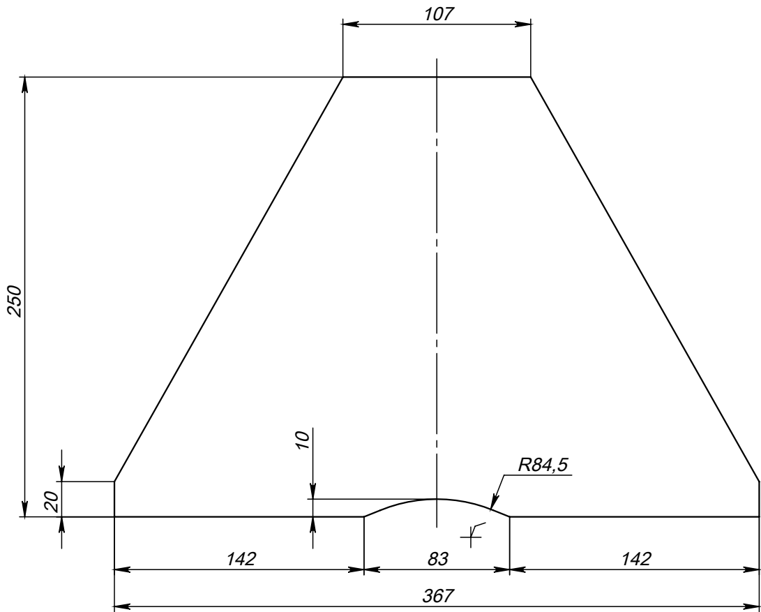
Поз.1 (Корпус) развертка
